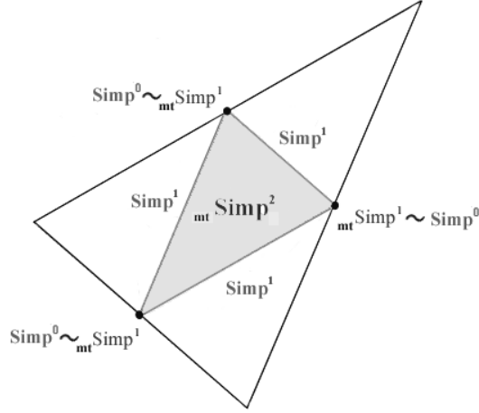
Рис. 1 Геометрическая структура двумерного срединно-усеченного симплекса
